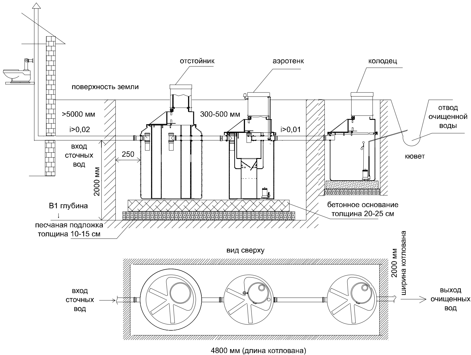
Рис. 6. Монтажная схема ЛОС со сборным колодцем
