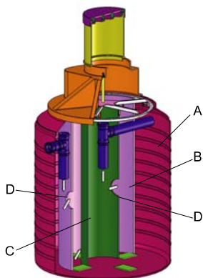
Рис. 3. Отстойник 3 м 3
