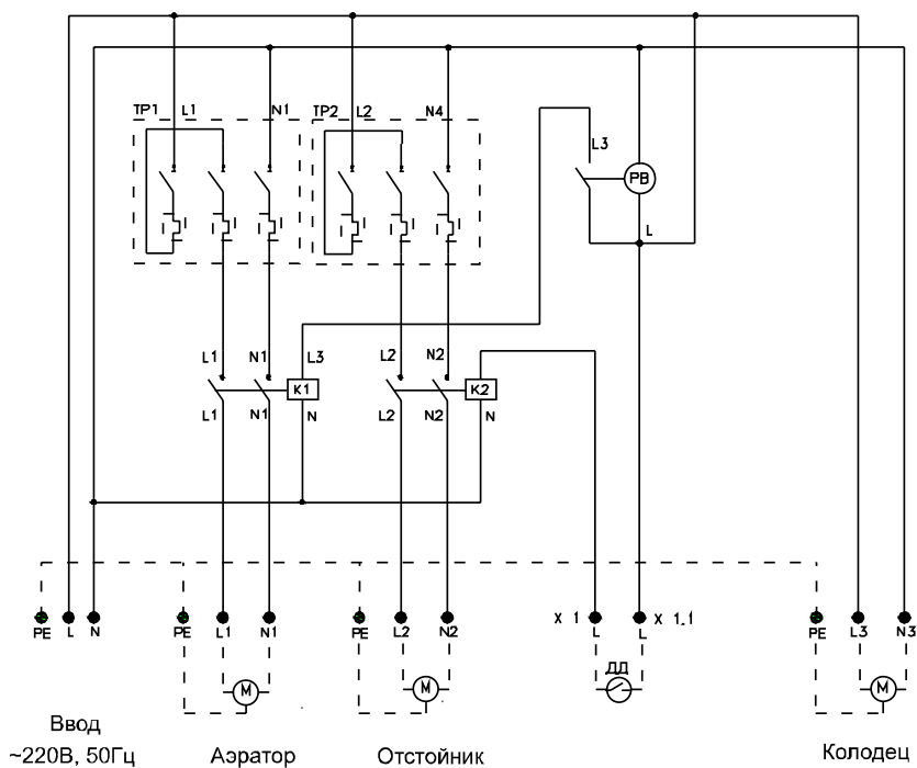
Рис. 7. Принципиальная схема щита управления ЛОС 5 и ЛОС 8
